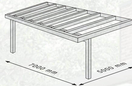
DIE ULTRALINE TERRASSENÜBERDACHUNG
