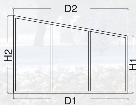
ANSICHT SEITENWAND MODELL TYP 2
