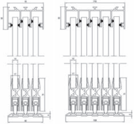
System AL22 untere Laufschiene, flach
