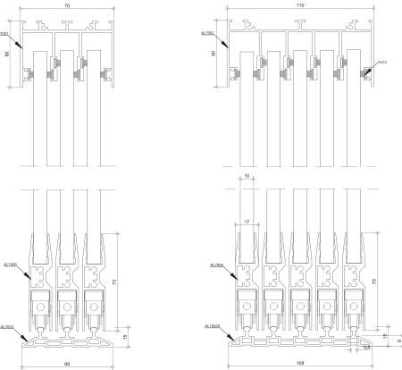
System AL24 Laufschiene durchgängig, hoch
