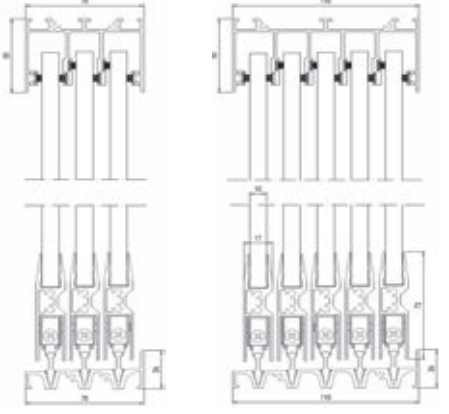
System AL23 untere Laufschiene, hoch
